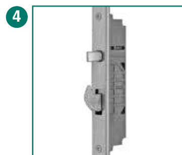
4 Sistema di chiusura tipo combi (rullo+gancio)
