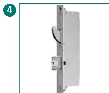
4 Chiavistello tipo gancio e chiavistello automatico che si chiudono in tandem
